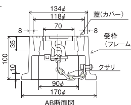
AB断面図
