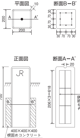
K2070JR (単位:mm)
