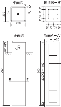
K2012JR (単位:mm)
