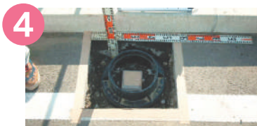
埋め戻し、ポイントホールの台座部分を設置する。
