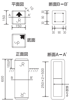
K1560JR (単位:mm)
